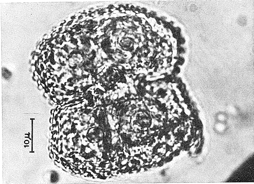
Fig. 1 - Cosmarium biretum Bréb.
