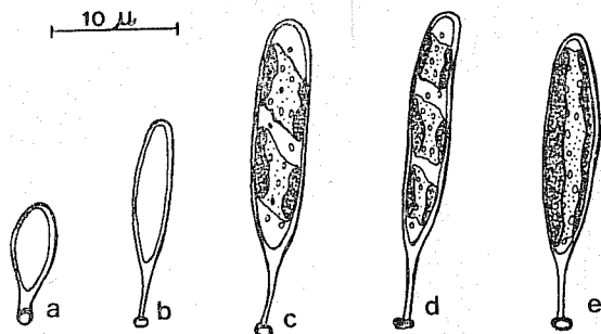
Fig. 2 - Characiopsis closteriana nov. sp.: a-b) stadi giovanili; c-d-e) stadi adulti dell'alga, con numero di cromatofori variabile da 1 a 3.
