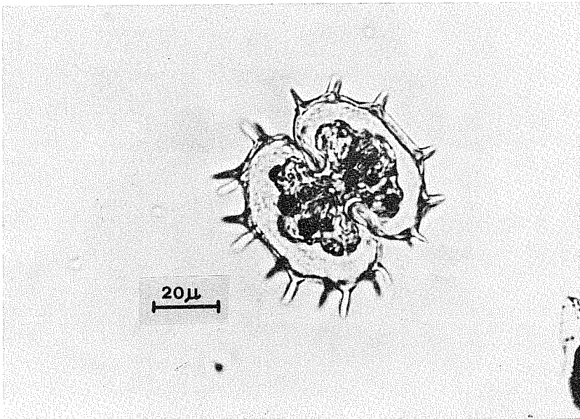
Fig. 2 - Xanthidium fasciculatum Ehr.
