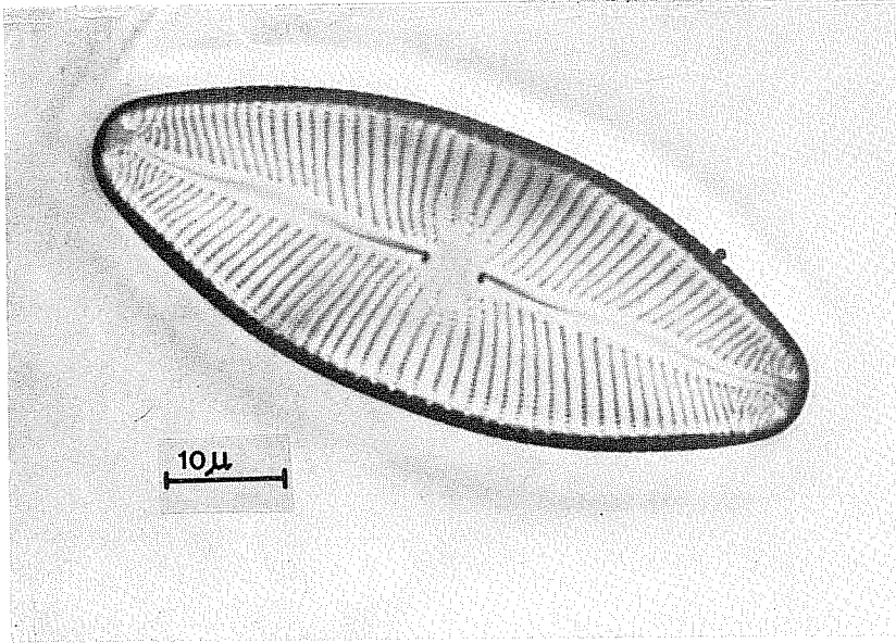
Fig. 1 - Navicula semen Ehr.
