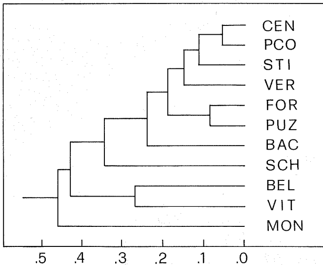
Fig. 4 - Dendrogramma illustrante i rapporti di similarità genetica tra dieci popolazioni di N. longicaudatus e una di N. pasquini .
