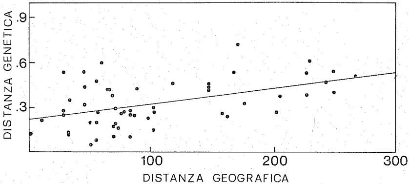
Fig. 3 - Relazione tra distanza genetica e distanza geografica per tutti i confronti tra coppie di popolazioni di N. longicaudatus e N. pasquini .
